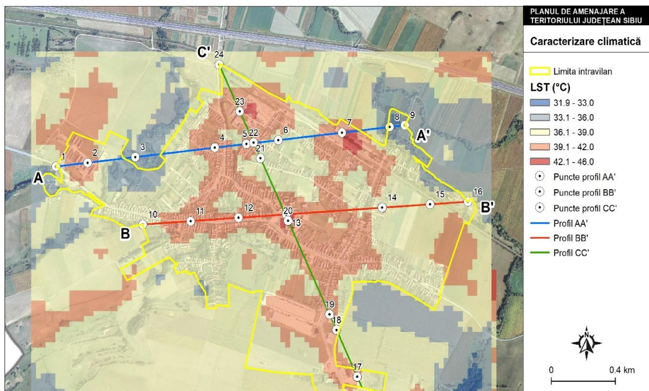
Fig. 2.93 HARTA TEMPERATURII SUPRAFEȚELOR ÎN ORAȘUL MIERCUREA SIBIULUI
