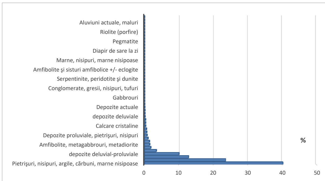
Fig. 2.24 DISTRIBUȚIA PROCENTUALĂ A CLASELOR PETROGRAFICE LA NIVELUL JUDEȚULUI
