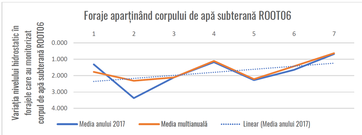
Fig. 2.45 EVOLUȚIA MEDIEI NIVELURILOR HIDROSTATICE MULTIANUALE ȘI A MEDIEI ANUALE PENTRU 2017 PENTRU CORPUL DE APĂ SUBTERANĂ ROOT06
