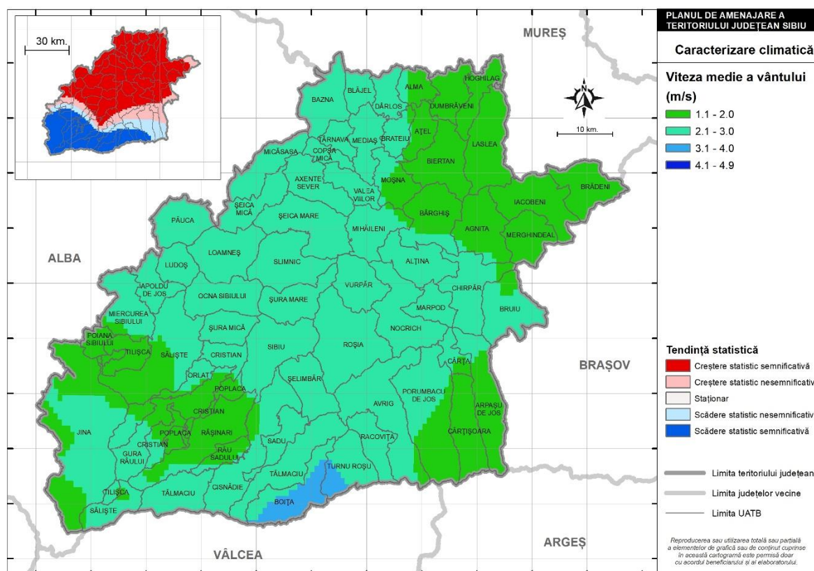
Fig. 2.16 VITEZA MEDIE MULTIANUALĂ A VÂNTULUI ÎN JUDEȚUL SIBIU ȘI TENDIŢA DE EVOLUȚIE PENTRU PERIOADA 1961-2021
