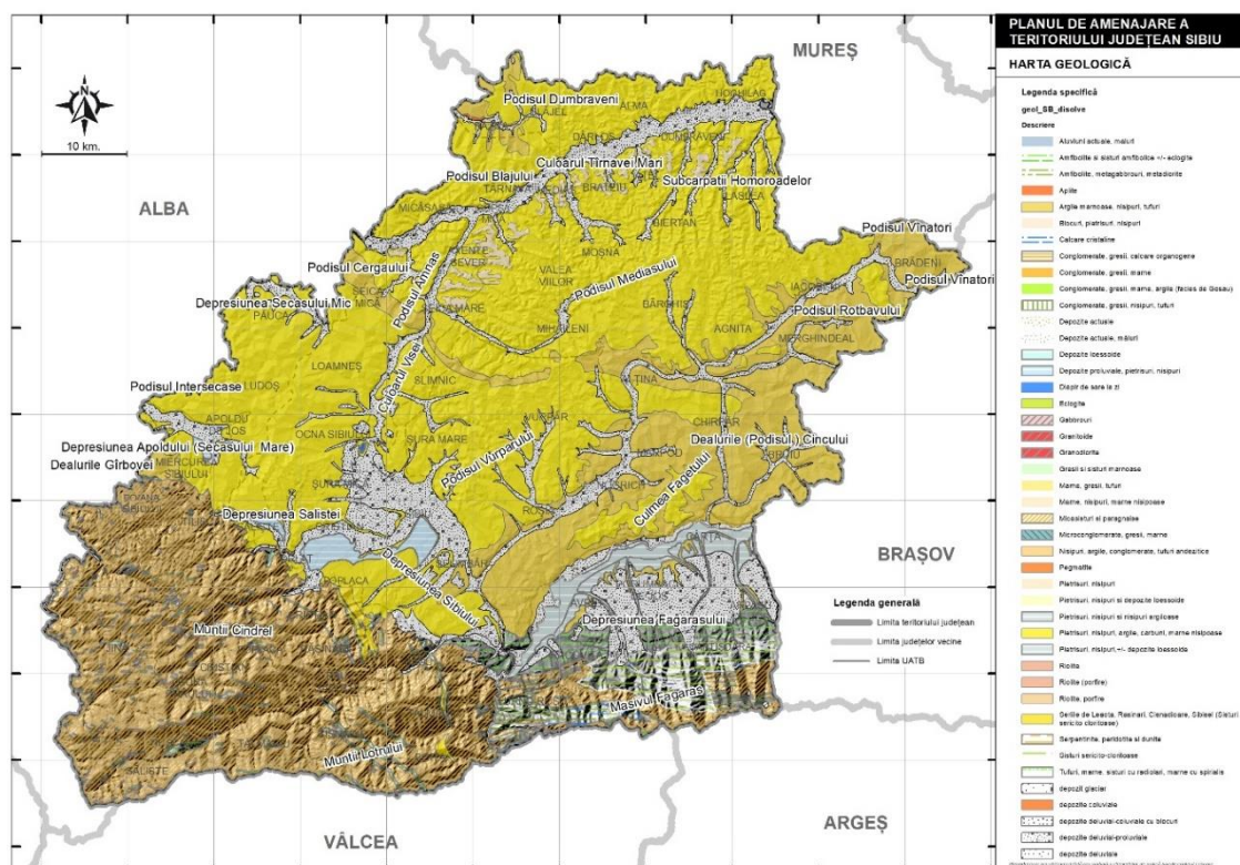
Fig. 2.23 HARTA GEOLOGICĂ
