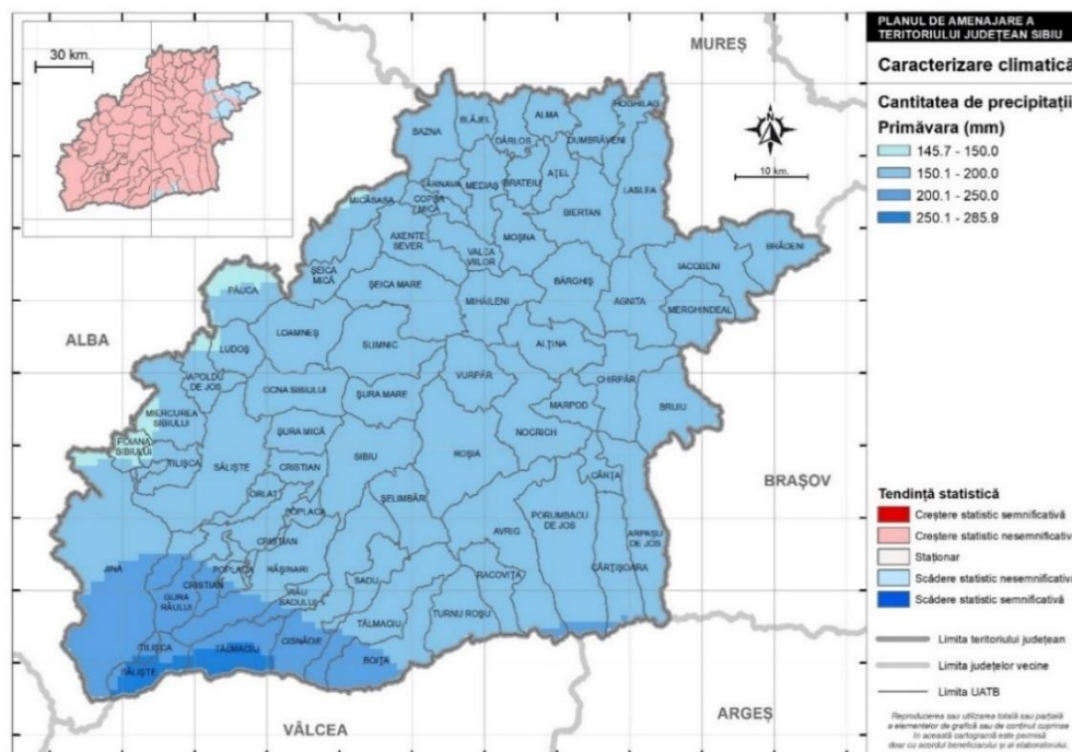
Fig. 2.9 CANTITATEA ANOTIMPUALĂ MEDIE MULTIANUALĂ DE PRECIPITAȚII PENTRU ANOTIMPUL DE PRIMĂVARĂ ÎN JUDEȚUL SIBIU ȘI TENDINȚA DE EVOLUȚIE PENTRU PERIOADA 1961-2021
