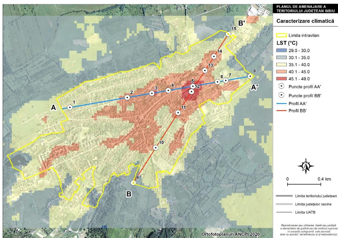
Fig. 2.84 HARTA TEMPERATURII SUPRAFEȚELOR ÎN ORAȘUL CISNĂDIE
