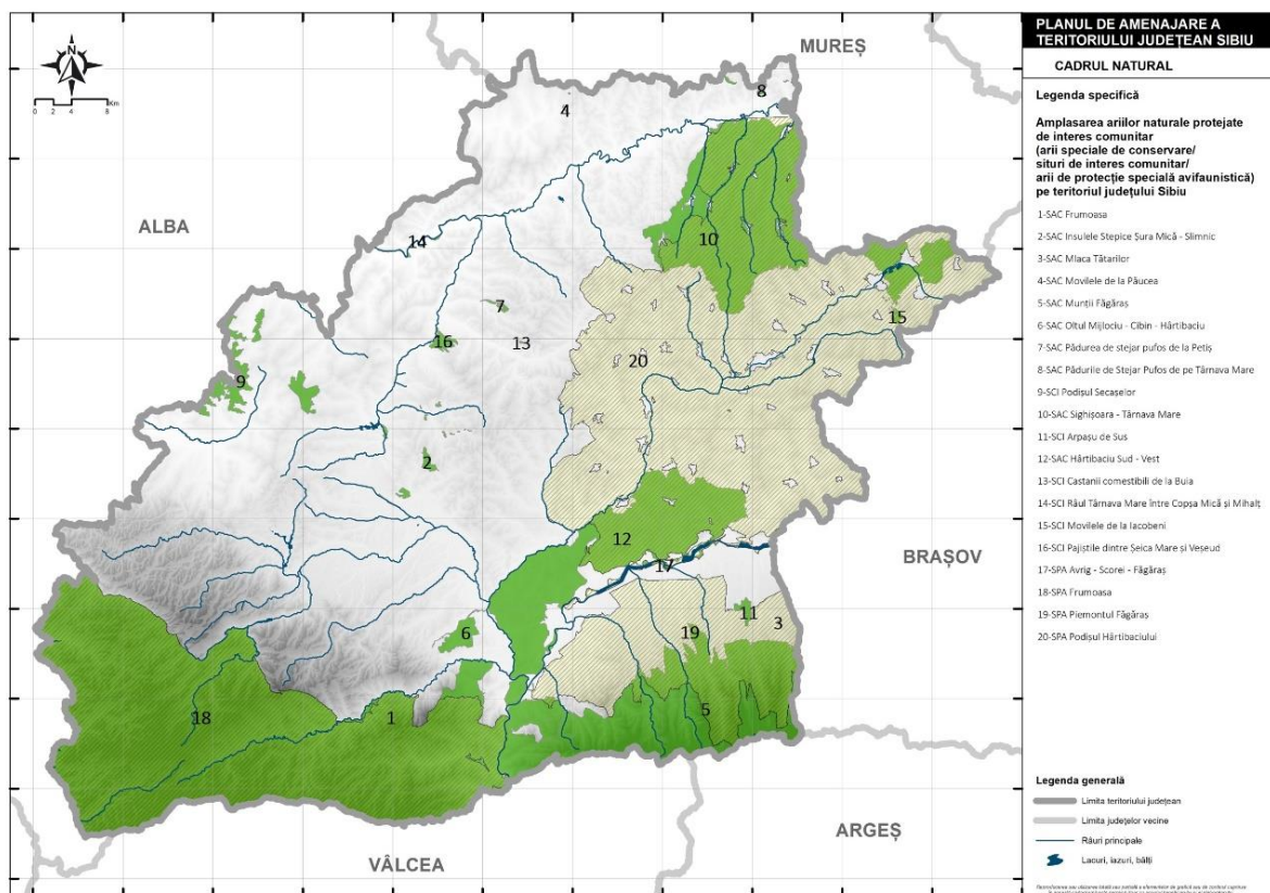
Fig. 2.33 DISTRIBUȚIA ARIILOR NATURALE PROTEJATE DIN REȚEAUA NATURA 2000 PE TERITORIUL JUDEȚULUI SIBIU
